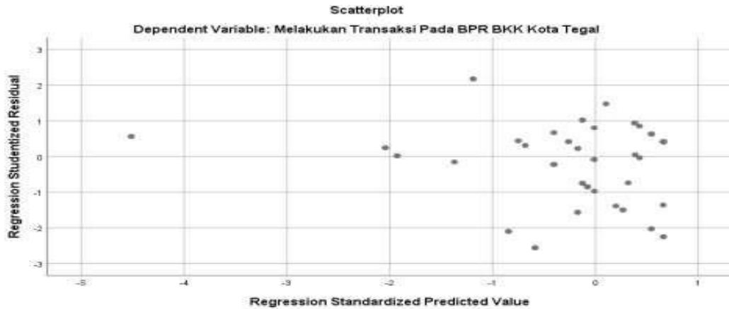
Gambar 4.3 Grafik Scatterplot
